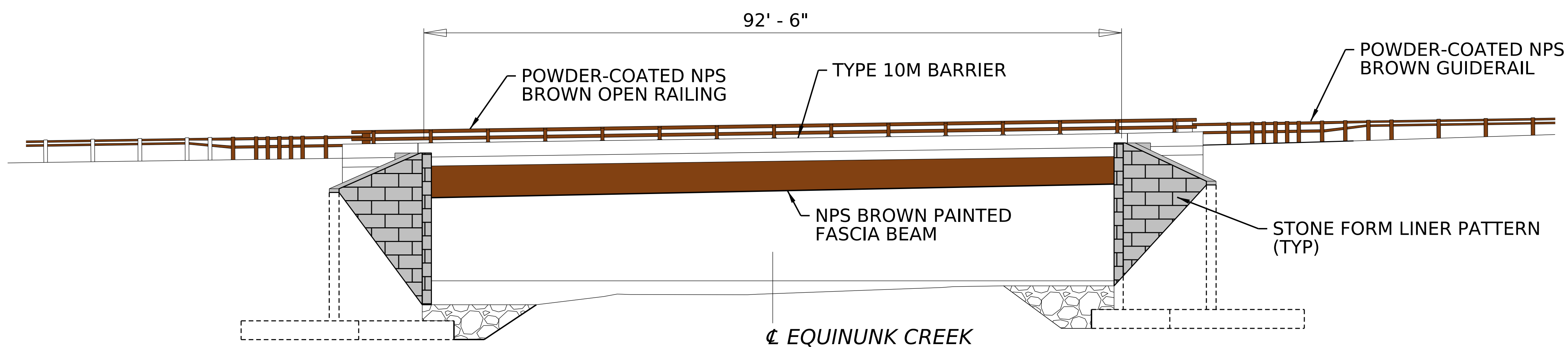
ELEVATION
